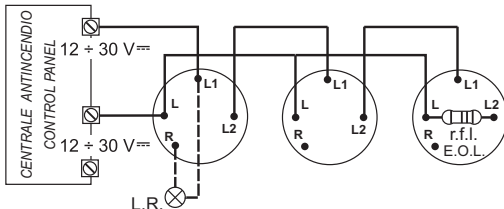
FIG. 8 Schema di Collegamento Semplificato con rilevatori serie 600 Simplified Circuit Diagram with the 600 series of detectors
