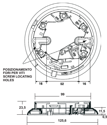
FIG.1 Dimensioni fissaggio per Base Rilevatore Fixing Dimensions for Detector Base
