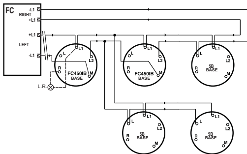
FIG. 7 Schema di Collegamento Semplificato con rilevatori serie FC400 Simplified Circuit Diagram with the FC400 series of detectors
